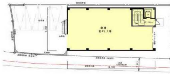
1階平面兼配置図
