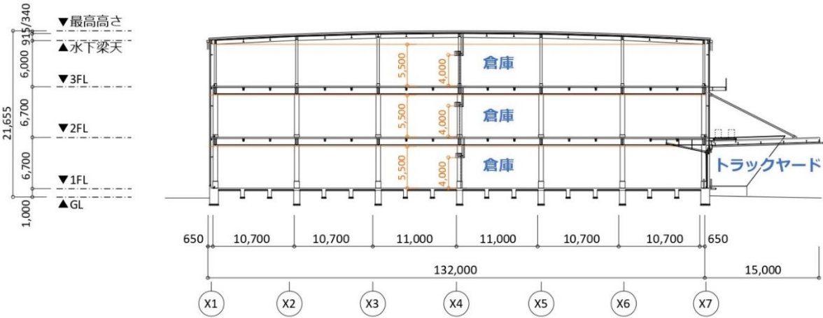
A-A 断面図
