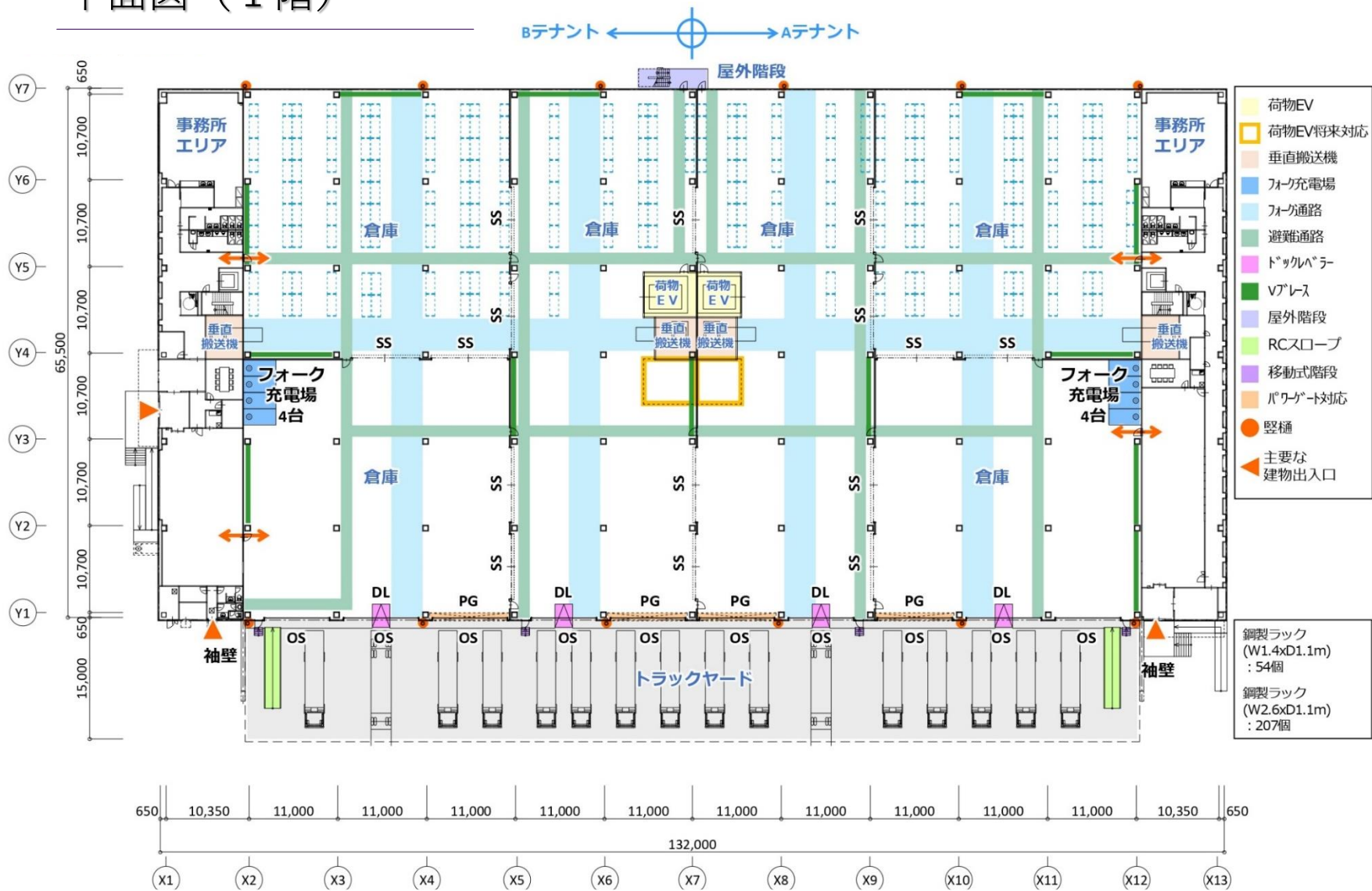
平面図（1階）
