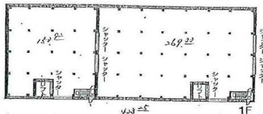
倉庫図面
