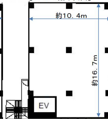
【4.5.6階平面図】
