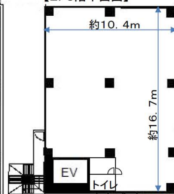
【2.3階平面図】
