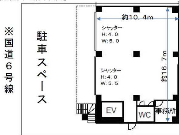
【配置図・1階平面図】
