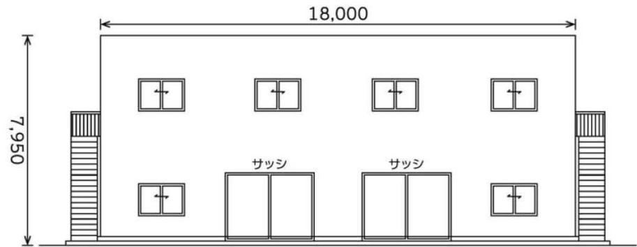
西側立面図
