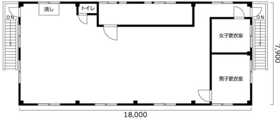
2階平面図
