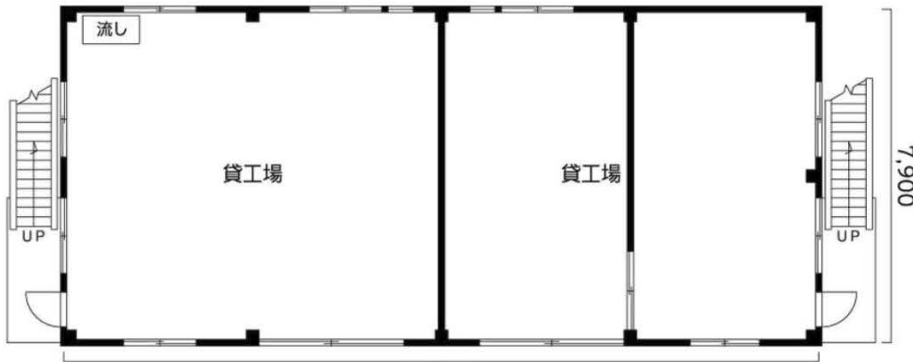
1階平面図
