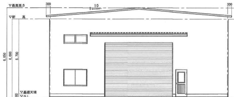
【正面側立面図】
