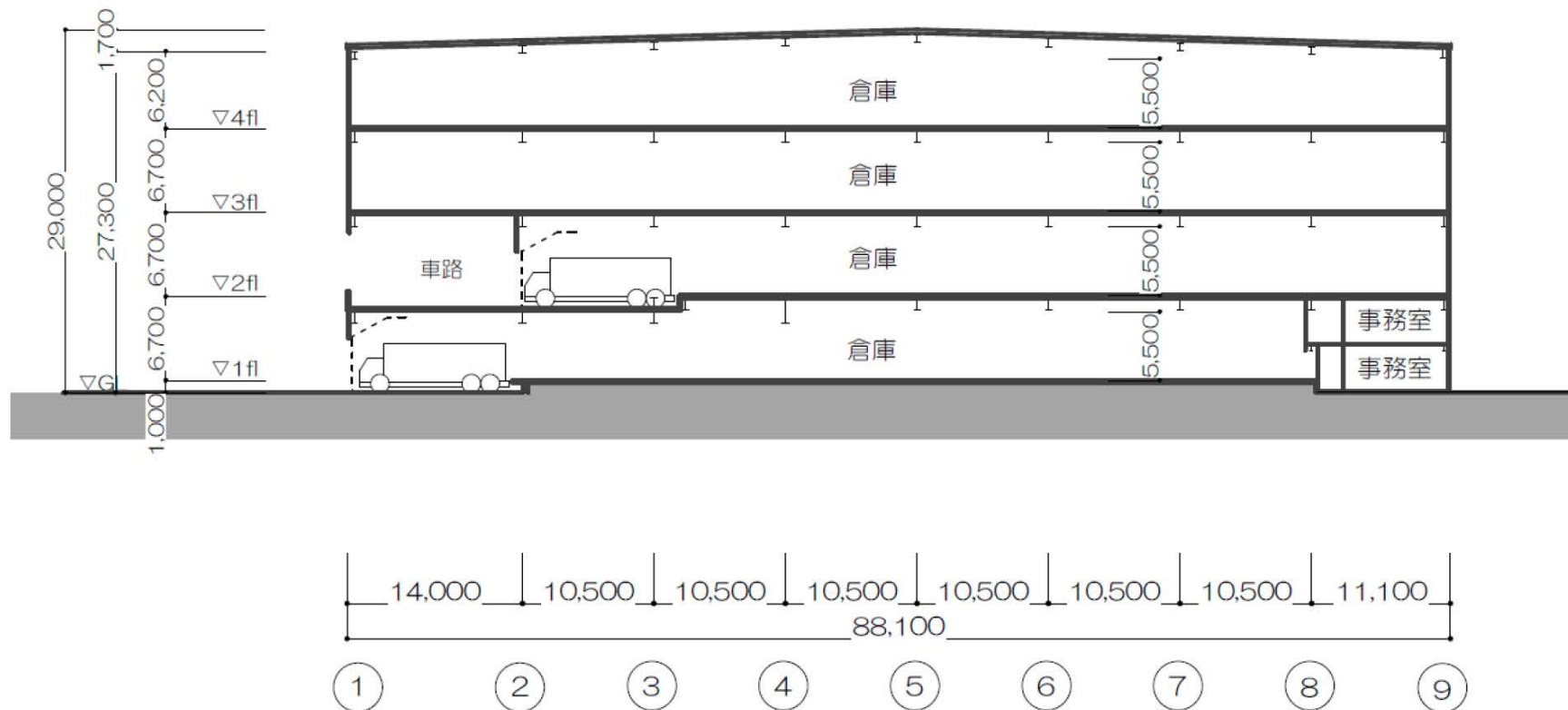
断面図
