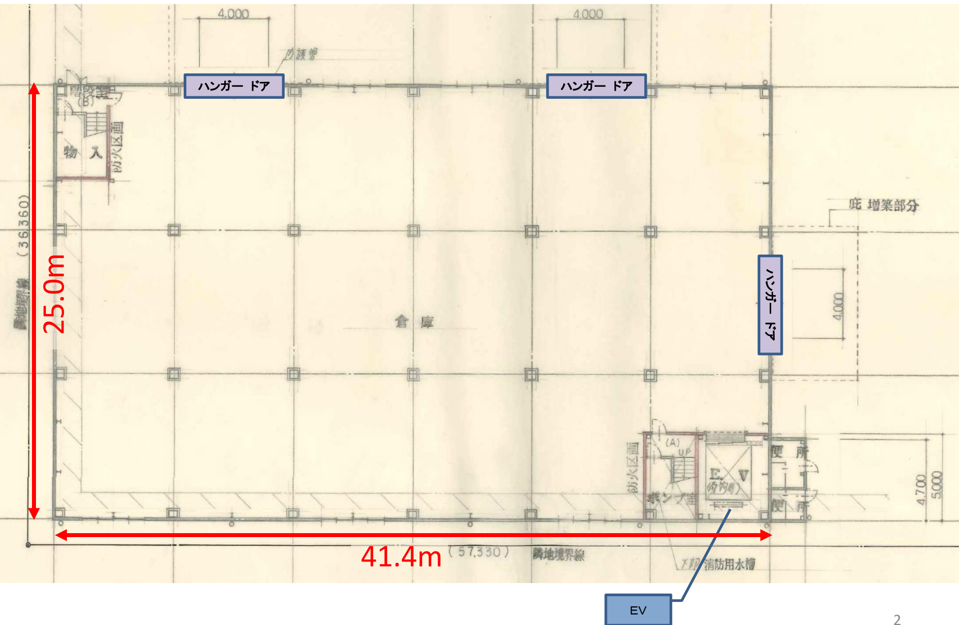
【1F 平面図】
