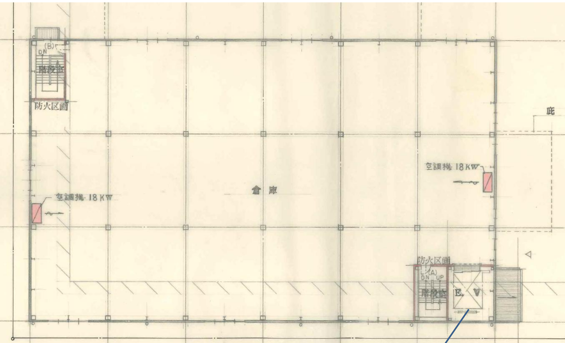
【2F 平面図】
