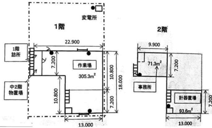
間取図
