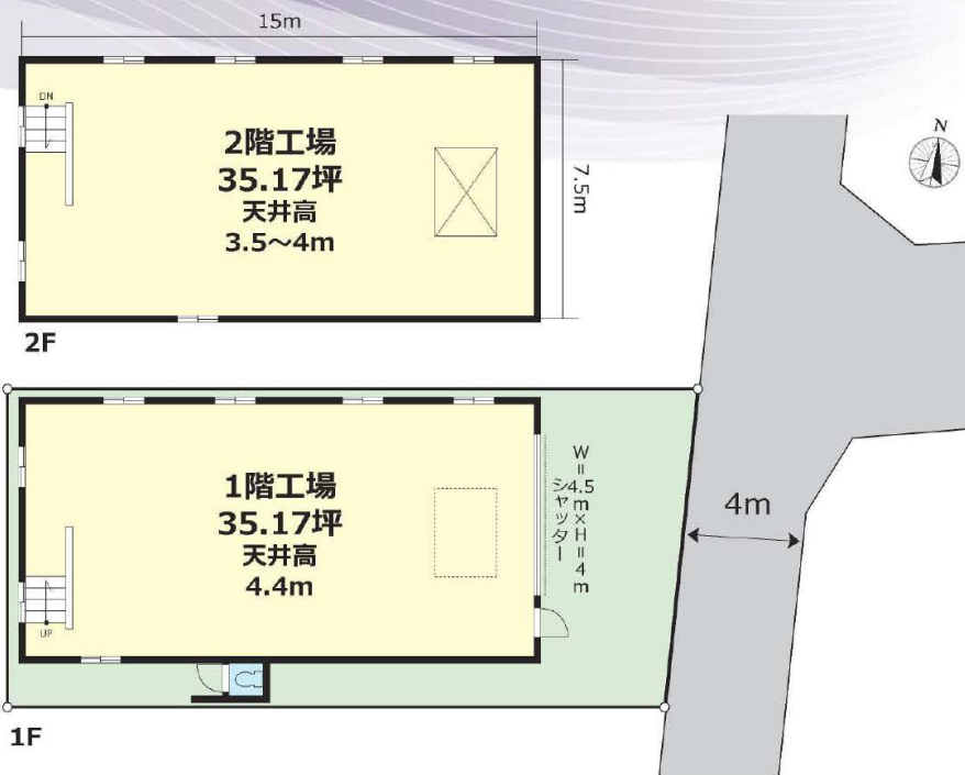
1階工場
