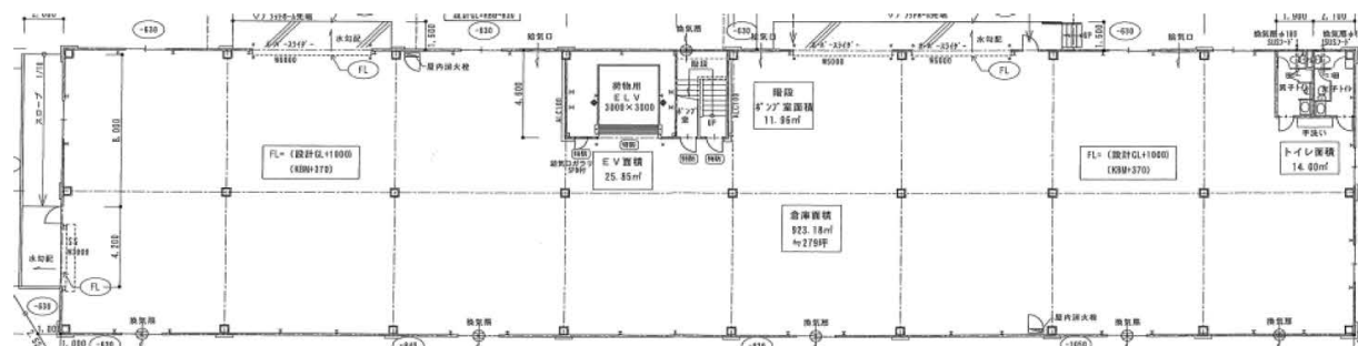
【1階平面図】
