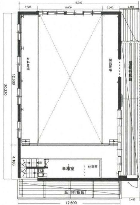
(2階平面図)
