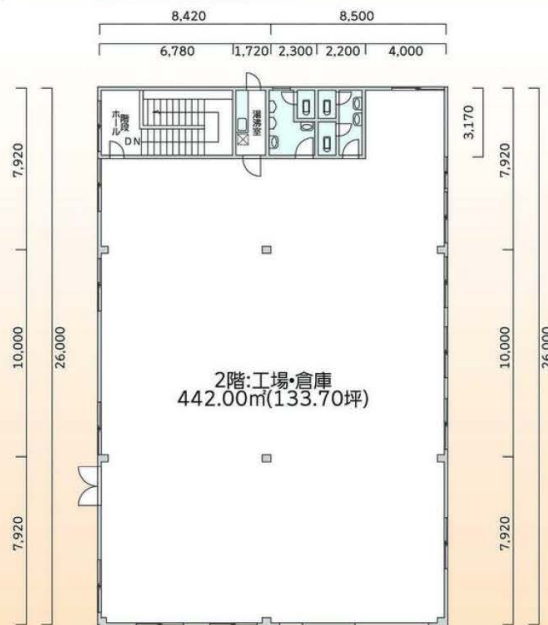
2階平面図
