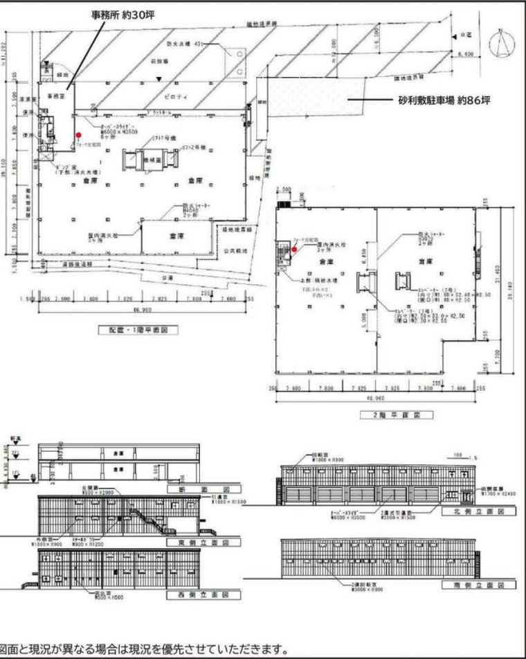
配置図・平面図
