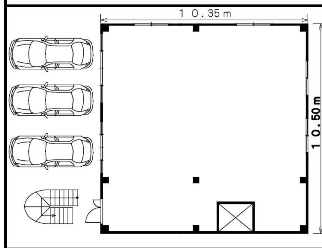
1階平面図 108.67㎡ (32.87坪)
