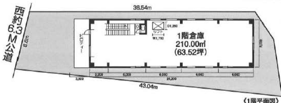
《1階平面図》
