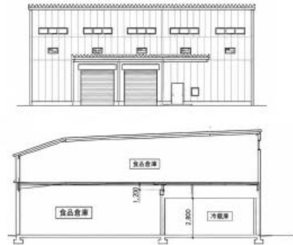
立面図・断面図
