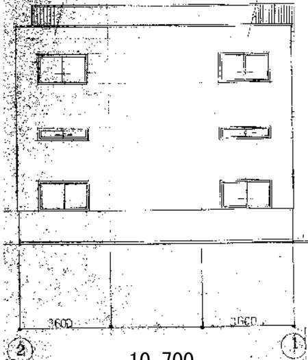
北側立面图 1/100
