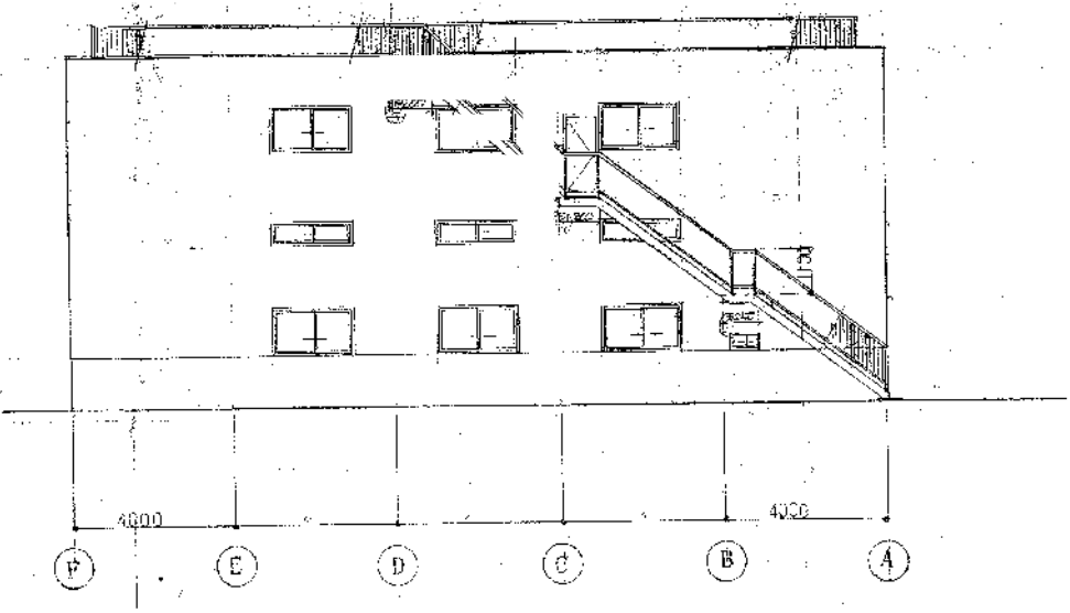
東立面图
