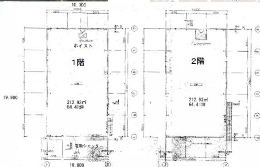
【平面図】
