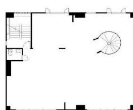
2階平面図
