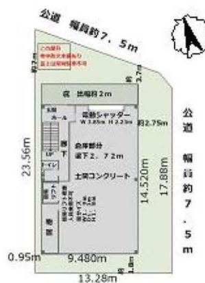
敷地及び一階平面図
