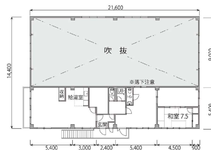
2階平面図
