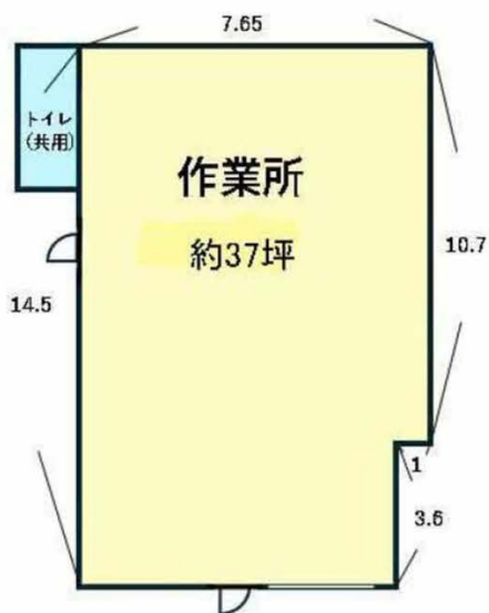
《平面図》
