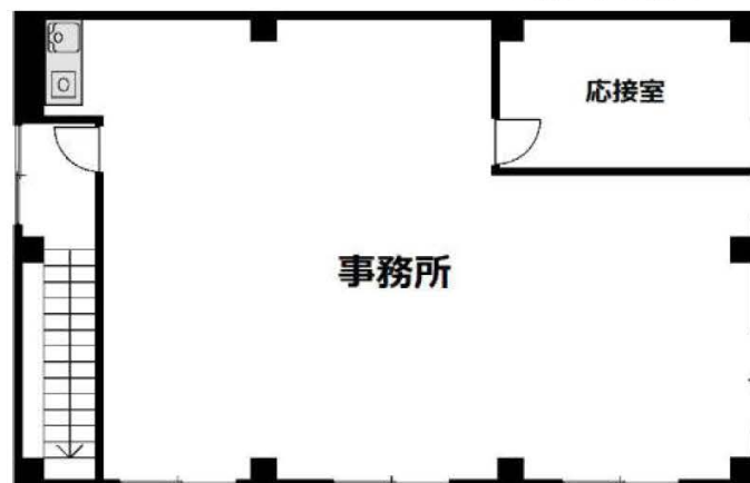
2階平面図
