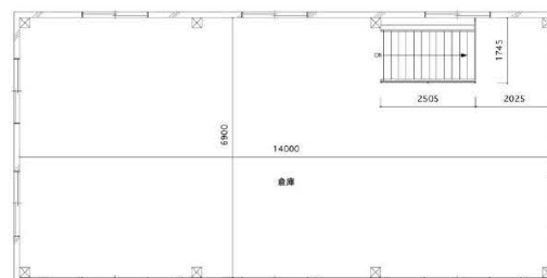
2階図面
