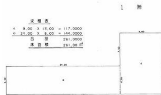
<1階間取り図>
